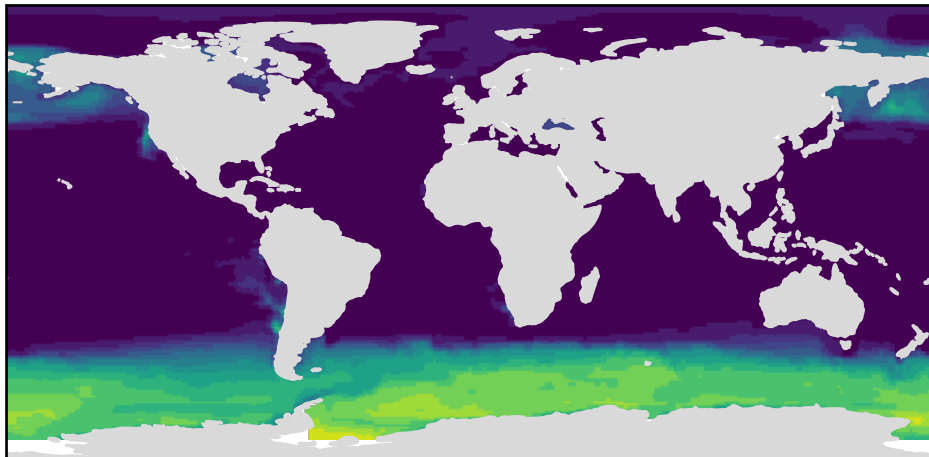
(a) HadGEM2-ES (r1i1p1) surface nitrate 2005
