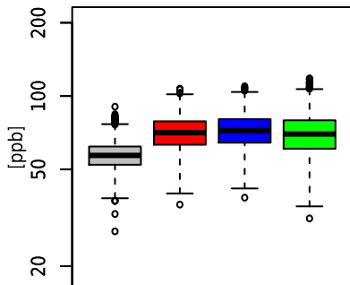
(d) Midwestern US
