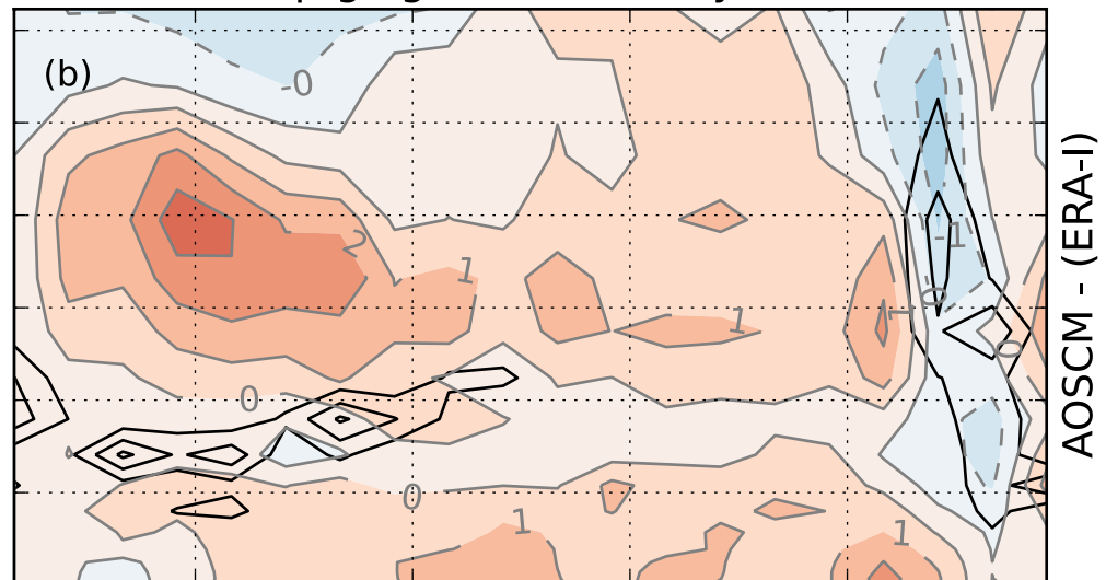
(b): q [ g\ kg^{-1} ], (d) salinity [PSU]
