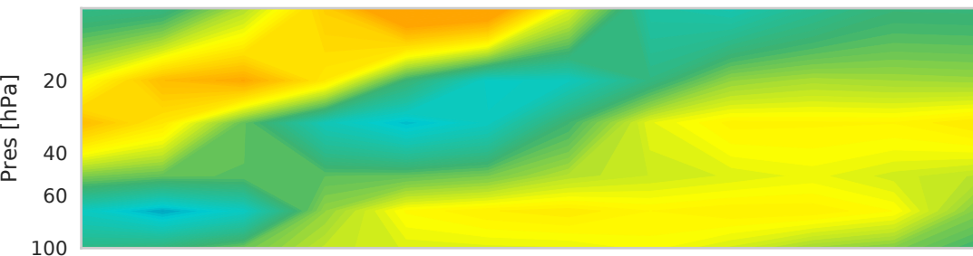
ERA-INTERIM
