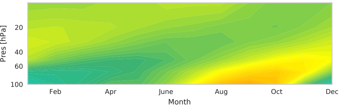
ERA-INTERIM
