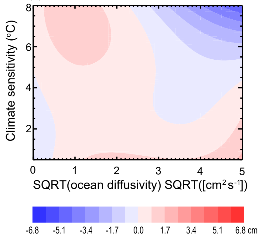
(d) thermosteric sea level rise
