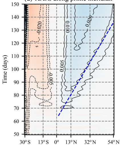
(d) IDEG along prime meridian
