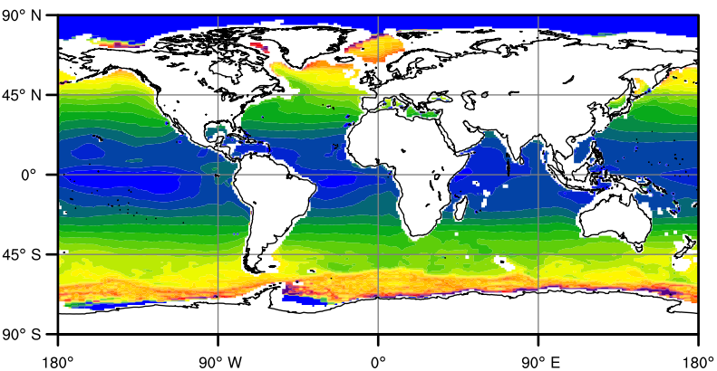
(b) Model LMDZ-old
