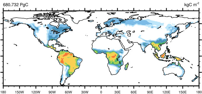
S_{\text{Clim,CO2}} C_{\text{veg}} JULES-C2
