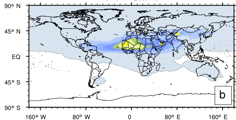
ICAP-MME : dust AOT
