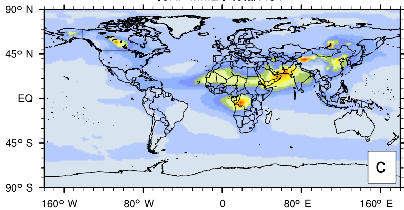
ICAP-MME : total AOT
