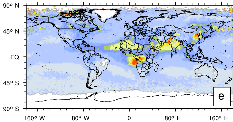
MODIS : total AOT
