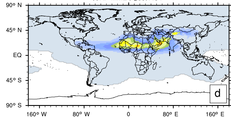
MODIS : total AOT
