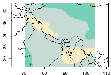
(d) ERA-Interim Feb meridional wind
