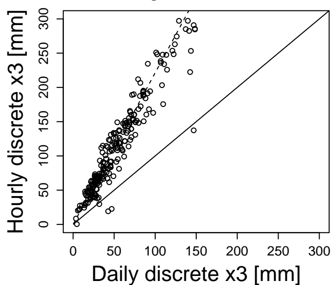
x3 parameter
