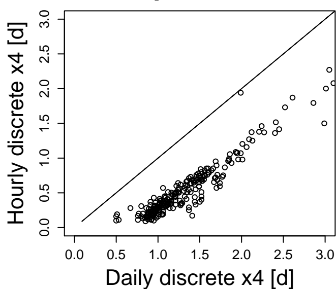
x4 parameter
