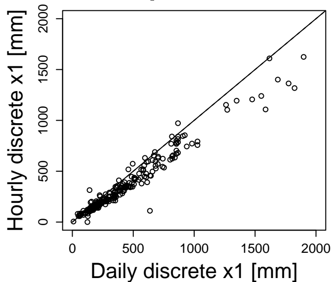
x1 parameter
