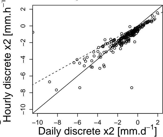
x2 parameter
